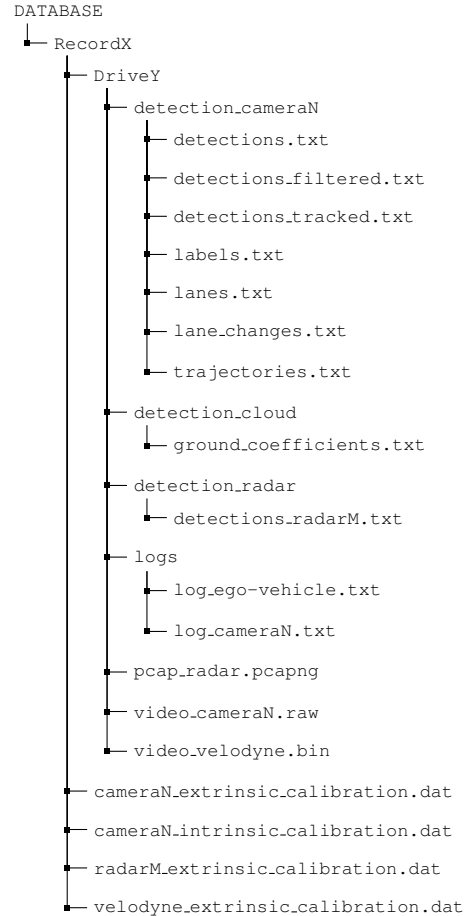
Fig. 3. Dataset Format.
